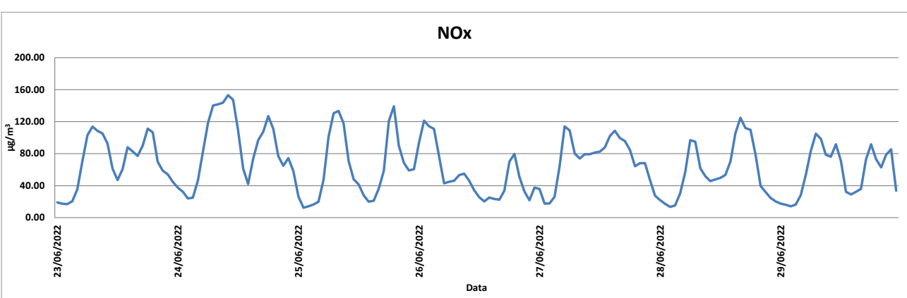
Grafico andamento media oraria del NO x in µg/m³
