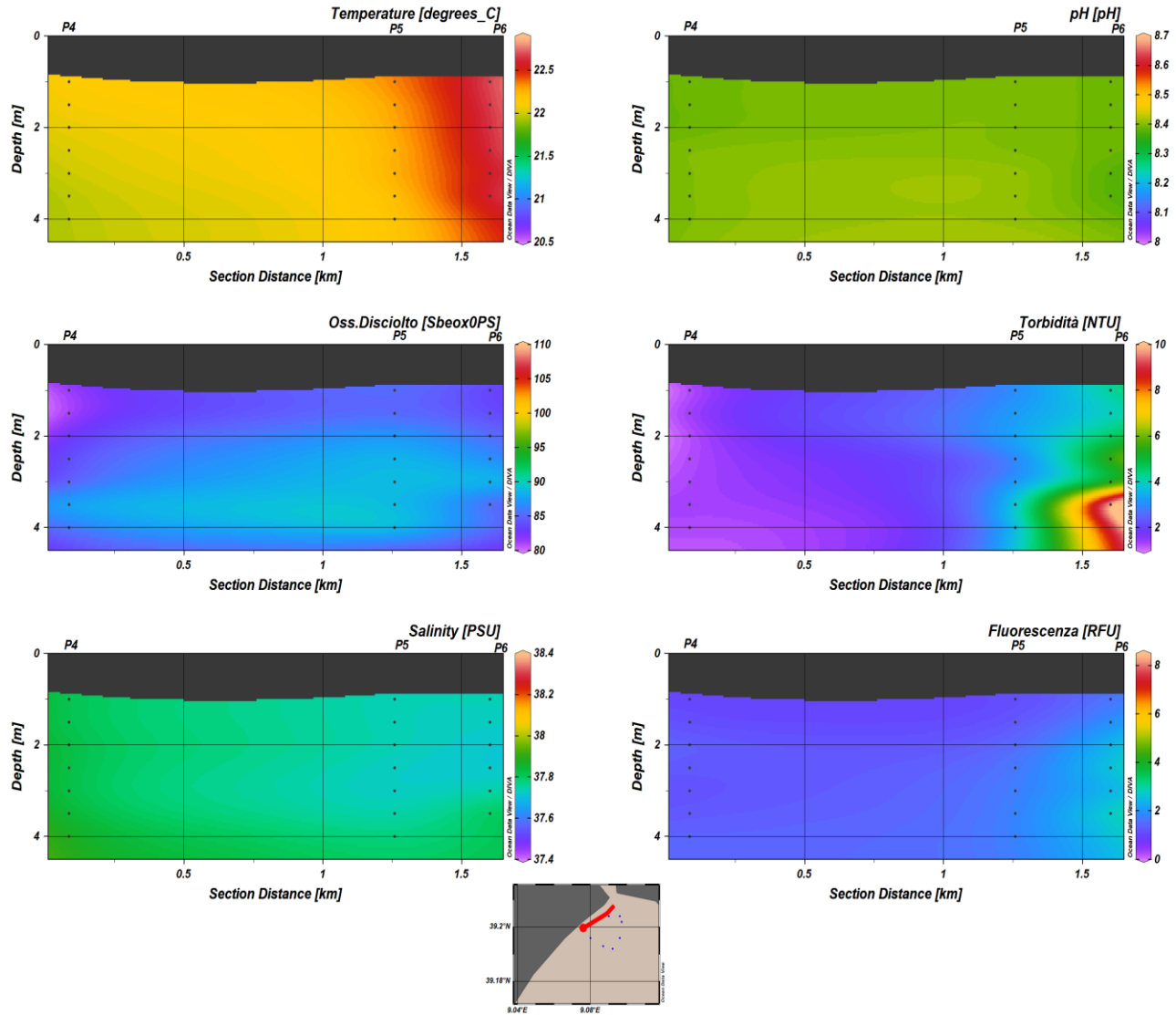
Fig.10 - Distribuzione spaziale della Temperatura, pH, Salinità, Torbidità, Clorofilla e % Saturazione.
