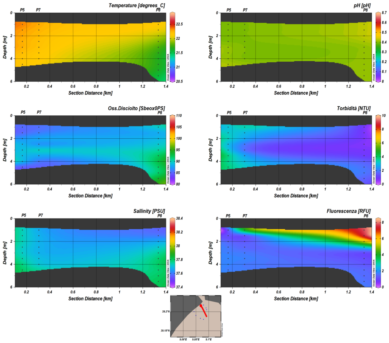
Fig. 11 – Distribuzione spaziale della Temperatura, pH, Salinità, Torbidità, Clorofilla e % Saturazione.
