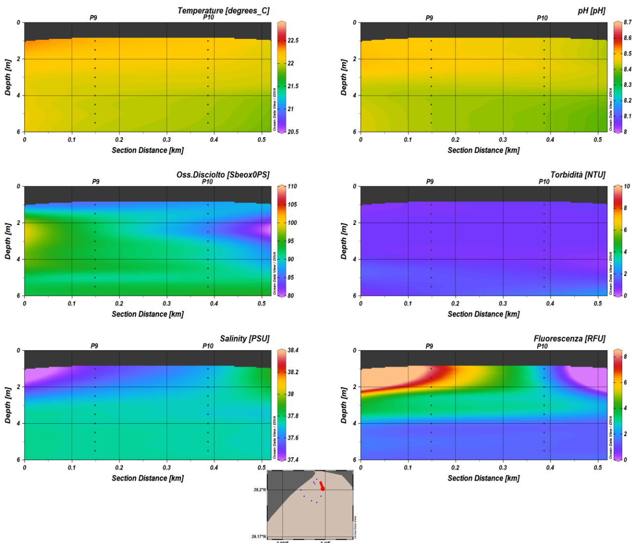
Fig. 12 - Distribuzione spaziale della Temperatura, pH, Salinità, Torbidità, Clorofilla e % Saturazione.
