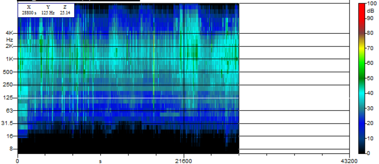
RLD4_notturmo - 1/3 Leq Spectrum + SLM - A
