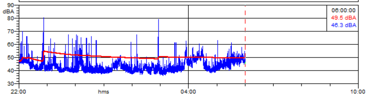
RLD4_notturmo - 1/3 Leq Spectrum + SLM - A
